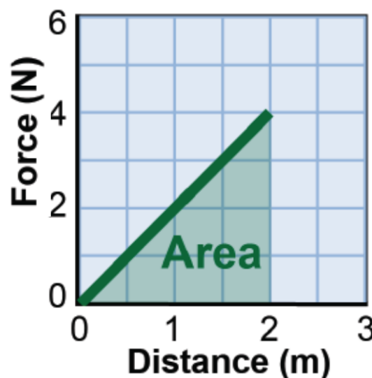
Figur 5.3: Lineært voksende kraft F = kx : W = \frac{1}{2} k x^2 er arealet av trekanten under kurven.
