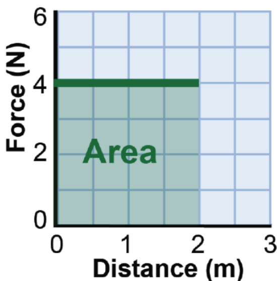
Figur 5.2: Konstant kraft: W = F \cdot s er arealet av rektangelet under kurven.
